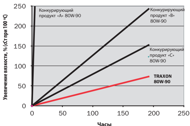
Испытание на окисляемость DKA (CEC-L-48-A-95) (192 часа при 160 °C) GL-5 80W-90
