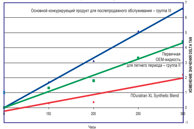
Испытание на окисляемость в алюминиевом стакане – АВОТ (Delta TAN) жидкость Duratran XL Synthetic Blend по сравнению с основным конкурирующим продуктом JDM J20C Summer и продукцией конкурентов для послепродажного обслуживания
